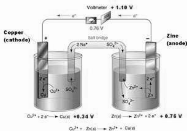
Малюнок 1. Гальванічний елемент Якобі-Данієля.
