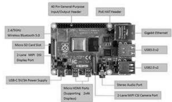
Рисунок 2 – Зовнішній вид та перелік інтерфейсів взаємодії Raspberry Pi 4 [5]
